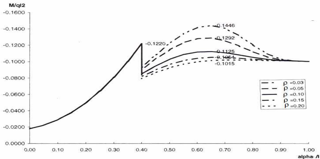
Fig VI.5. Variation du moment maximal sur appui
