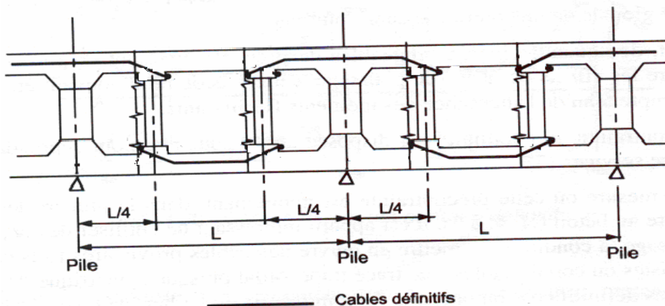
Fig.VIII.9. Disposition des câbles de poussage
