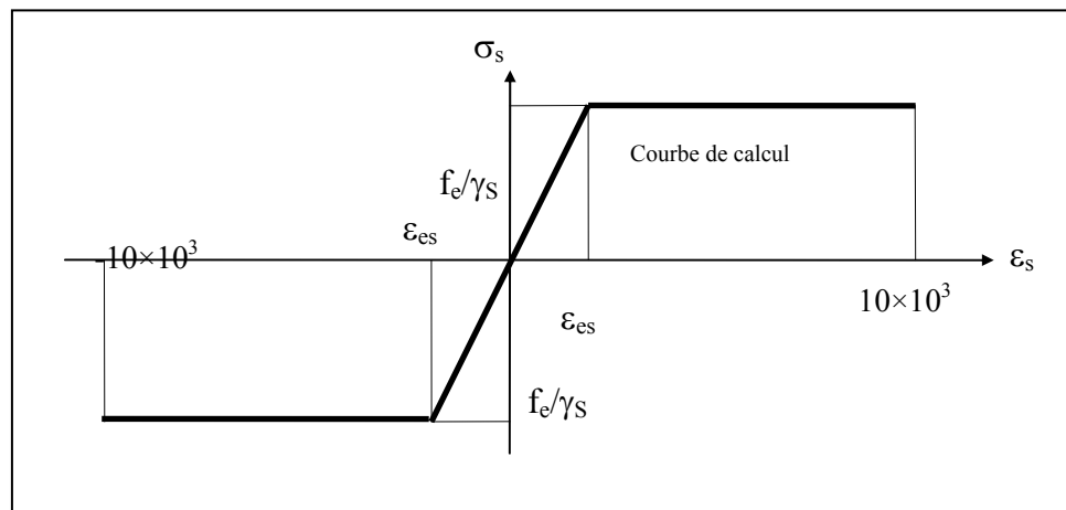
Fig.III.2. Diagramme contrainte-déformation.
