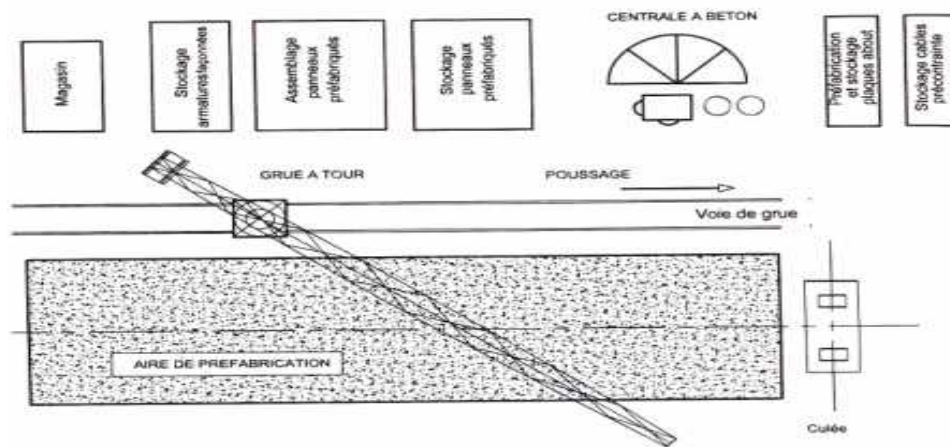
Fig.V.8.Instalation de préfabrication
