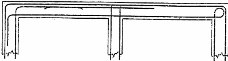
Fig. 9.2 Dispositions typiques des chaînages en plan
