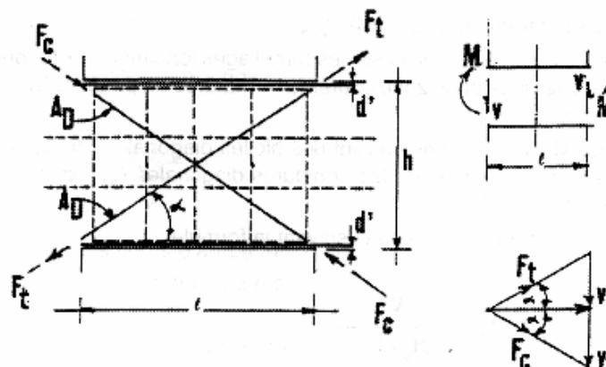
Fig.7.12 : Efforts dans les bielles du linteau
