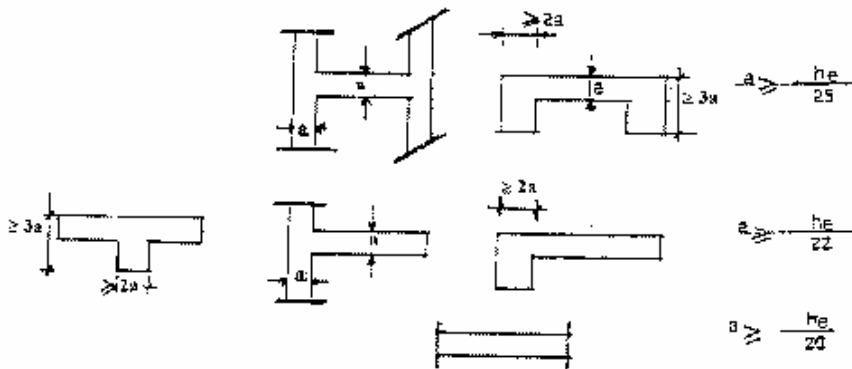
Fig. 7.8 : Coupes de voiles en plan
