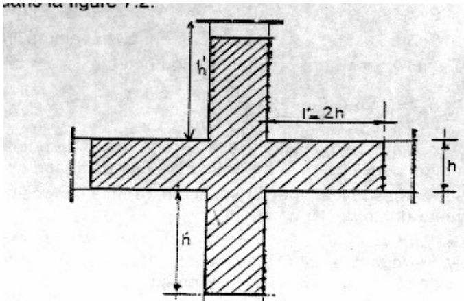
FIG. 7.2 : zone nodale
