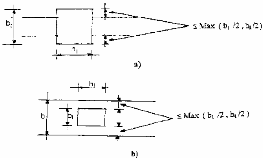
Fig 7.4 : Dimensions à respecter par les poutres
