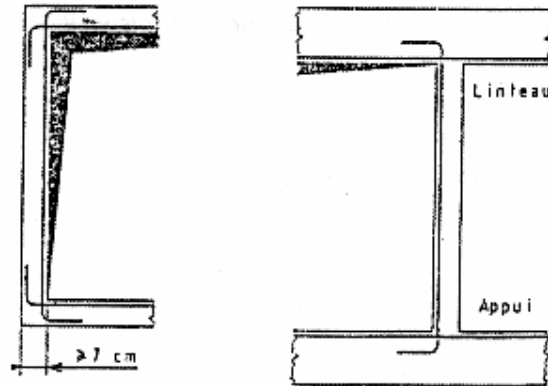
Encadrement en béton armé
