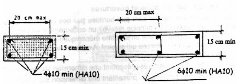
Fig. 9.3 chaînage des éléments structuraux
