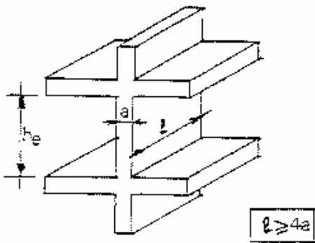
Fig. 7.7 : Coupe de voile en élévation
