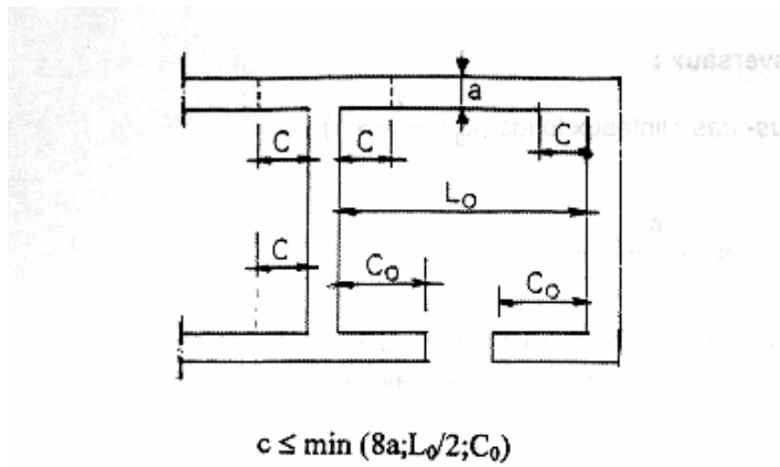
Fig. 7.9 : Prise en compte des murs en retour
