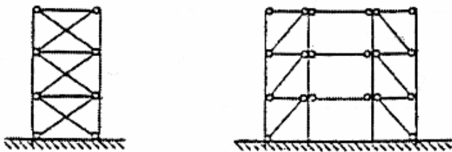
Fig. 8.1: Palées centrées en X
